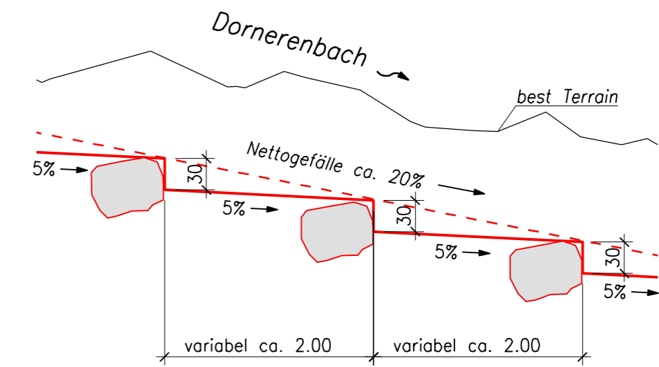
Sohlensicherung mit Steinschwellen Variante 1B
