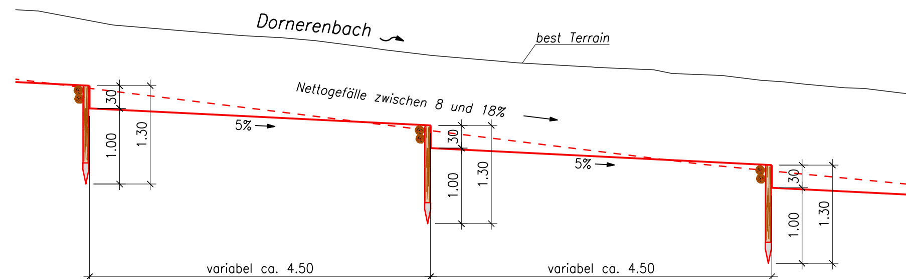
Sohlensicherung mit Holzschwellen Variante 2
