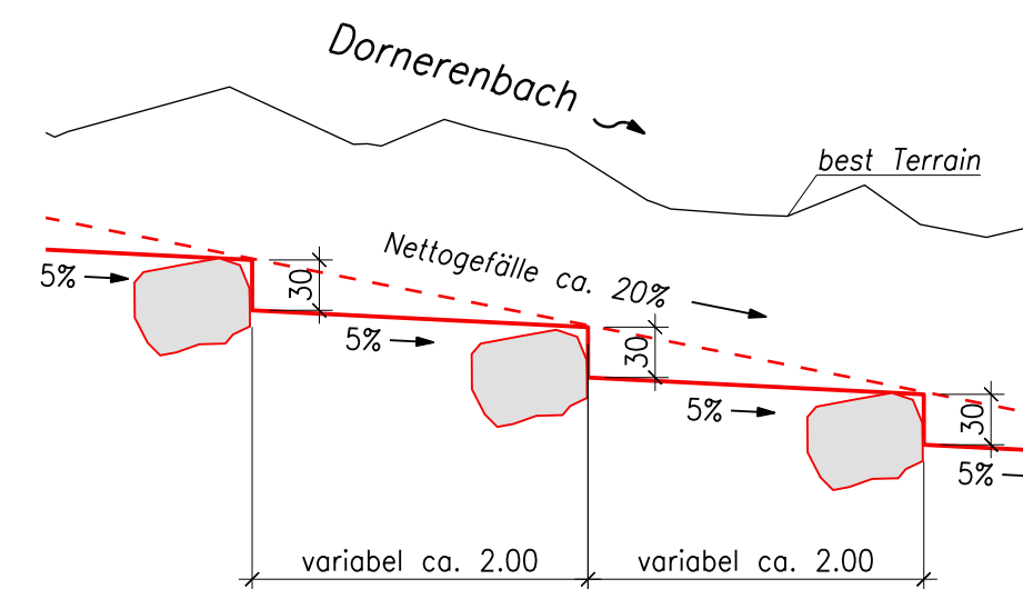
Sohlensicherung mit Steinschwellen Variante 1B
