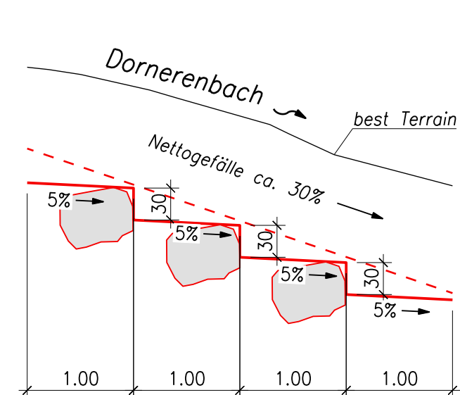
Sohlensicherung mit Steinschwellen Variante 1A
